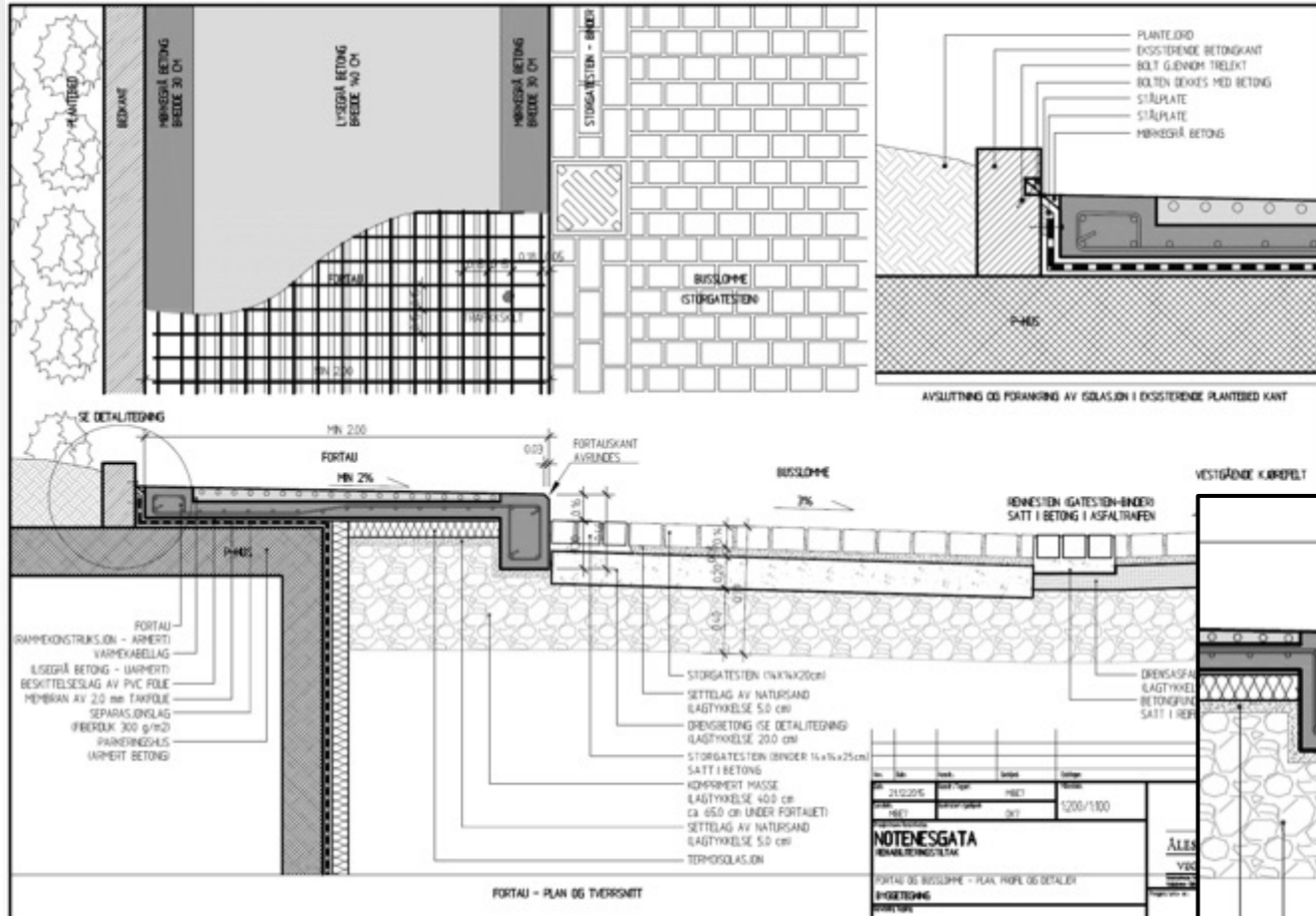
Bussholdeplass og P-hus - Prinsippdetaljer
